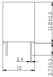
安装图
